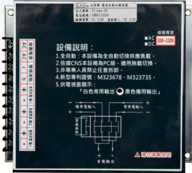
型 式：VC-hmv-20 外型尺寸：132長x167寬x76深mm 面板開孔：133長x137寬mm
