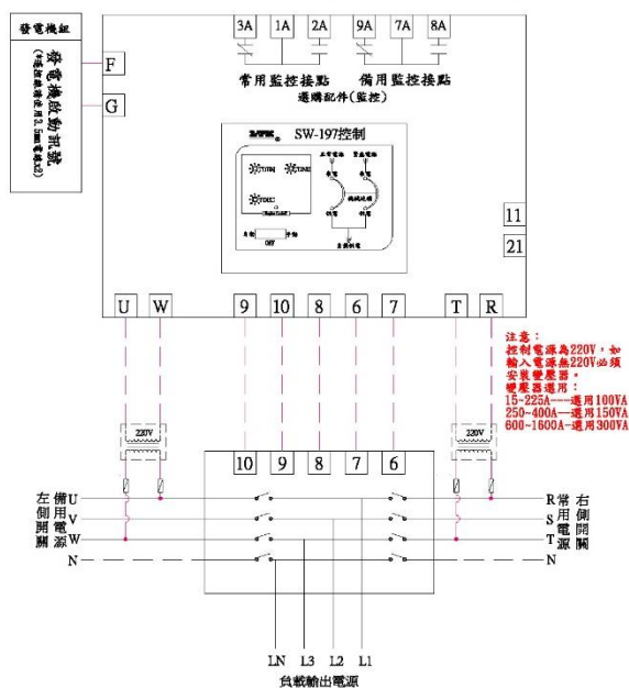
ATS. 右側(II路)優先供電配置圖
